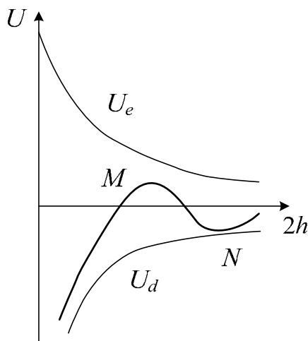
Рис. Изменение энергии ( U ) тонкой пленки электролита в зависимости от ее толщины ( h )
