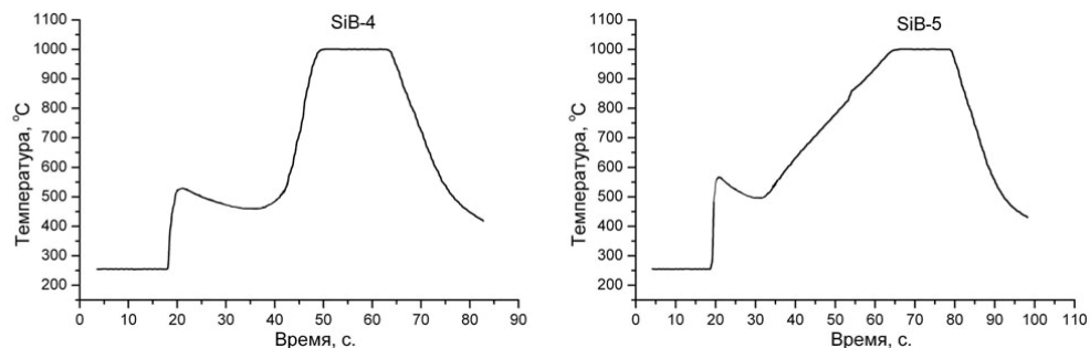
Рис.4. Графики зависимости температуры отжига пластин SiB-4 и SiB-5 от времени при БТО ( \Phi = 7 \cdot 10^{14} \text{ см}^{-2} ).
