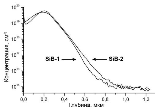
Рис. 6. Профили распределения бора в кремнии после БТО ( 1000^\circ\text{C} , 10 с). Имплантация дозой 1,5 \cdot 10^{15} \text{ см}^{-2} в один шаг (SiB-1) и дозой (1+2+4+8) \cdot 10^{14} \text{ см}^{-2} в четыре шага (SiB-2).
