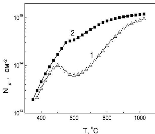
Рис.3. Кривые электрической активации имплантированного бора в слоях кремния: 1 – без подсветки электронами; 2 – с подсветкой электронами с энергией 10 кэВ при плотности тока электронов 5 мкА·см -2 .
