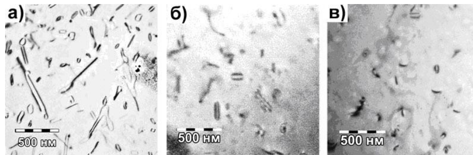
Рис. 5. ПЭМ фотографии слоев кремния, легированных бором: а – в один шаг дозой 7 \cdot 10^{14} \text{ см}^{-2} (SiB-3); б, в – в три шага дозой (1+2+4) \cdot 10^{14} \text{ см}^{-2} (SiB-4 и SiB-5). Отжиг БТО в течение 15 секунд при 1000^\circ\text{C} в \text{N}_2 .
